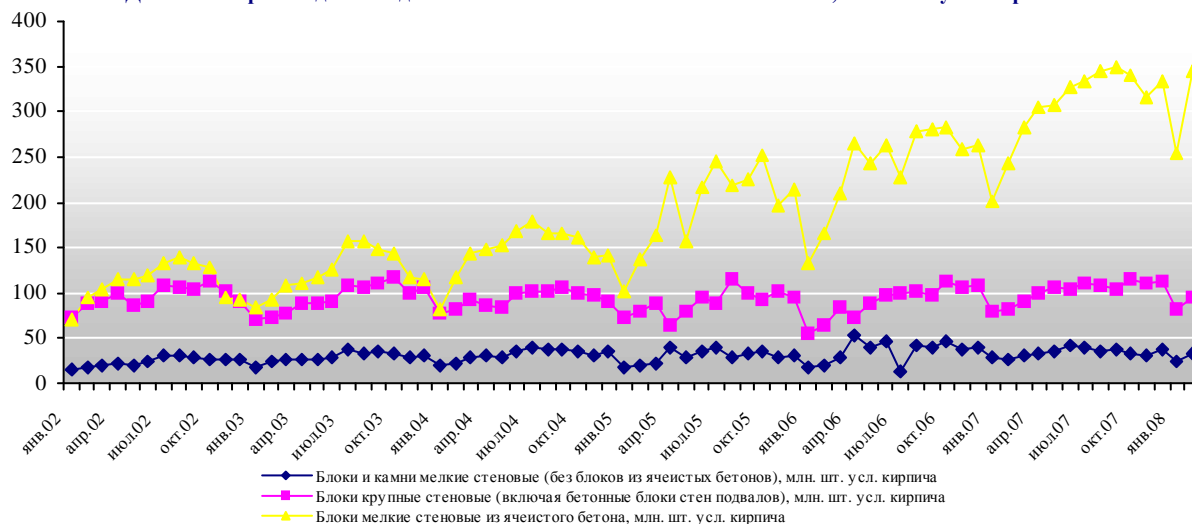
Производство изделий из бетона в России в январе-феврале 2007-2008гг.
