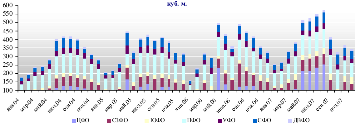
Динамика производства раствора в России по Федеральным округам в 2004-2007 гг., тыс. куб. м.
