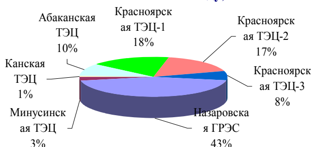
Структура установленных мощностей по электростанциям ОАО "ТГК-13" в 2012 году, МВт
