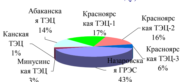
Структура установленных мощностей по электростанциям ОАО "ТГК-13" в 2014 году, МВт
