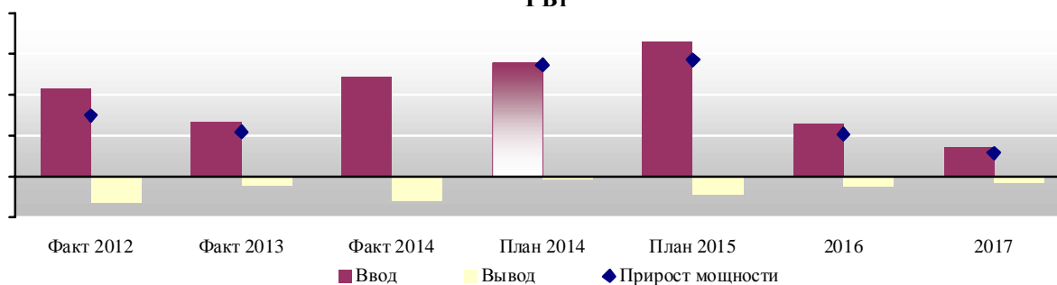
Изменение генерирующих мощностей в 2012-2014 гг. и прогноз до 2017 г., ГВт
