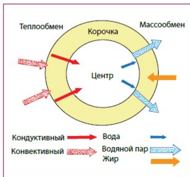
Рис. 2. Диаграмма тепло- и массообмена при обжаривании во фритюре (Bouchon, 2009)
