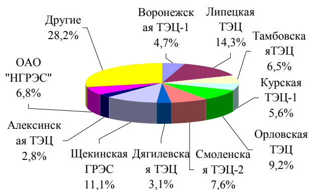
Структура установленных мощностей по электростанциям ОАО "Квадра" в 2012 году, МВт
