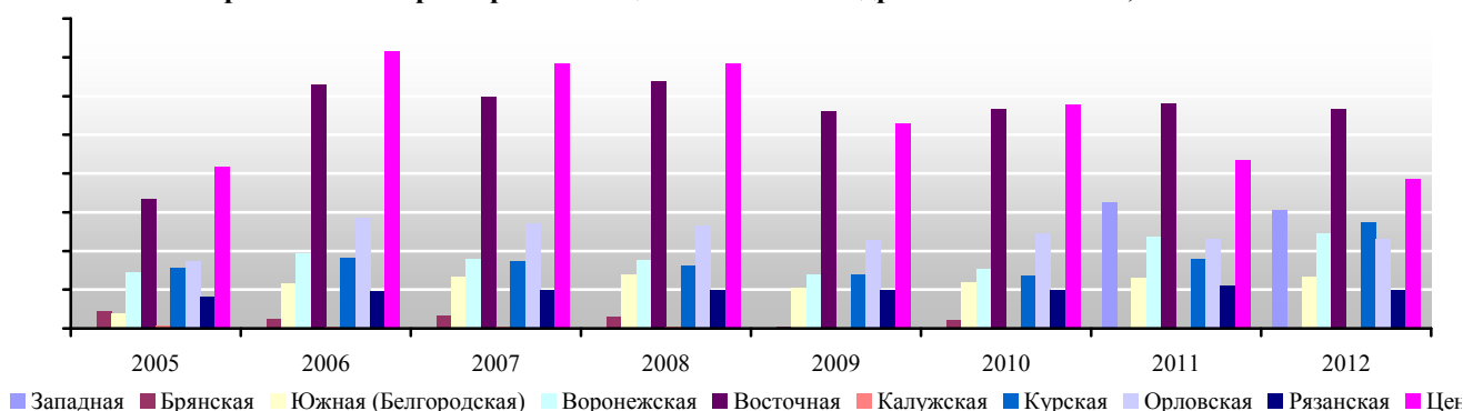
Выработка электроэнергии станциями ОАО "Квадра" в 2005-2012 гг., млн. кВт.ч
