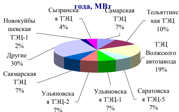
Структура установленных мощностей по электростанциям ОАО "Волжская ТГК" в начале 2013 года, МВт
