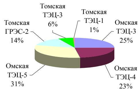
Структура установленных мощностей по электростанциям ОАО "ТГК-11" в 2015 году, МВт
