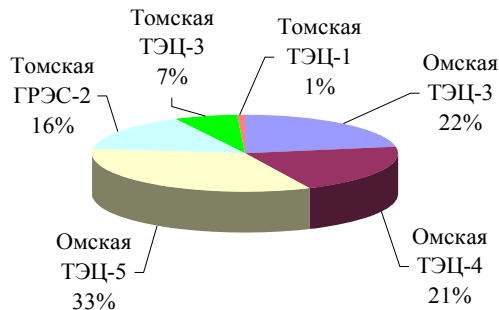
Структура установленных мощностей по электростанциям ОАО "ТГК-11" в 2013 году, МВт
