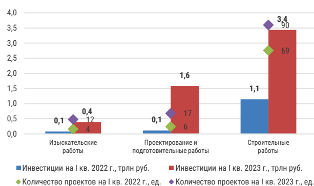
Распределение инвестиционных проектов в транспортировке нефти и газа по стадиям
